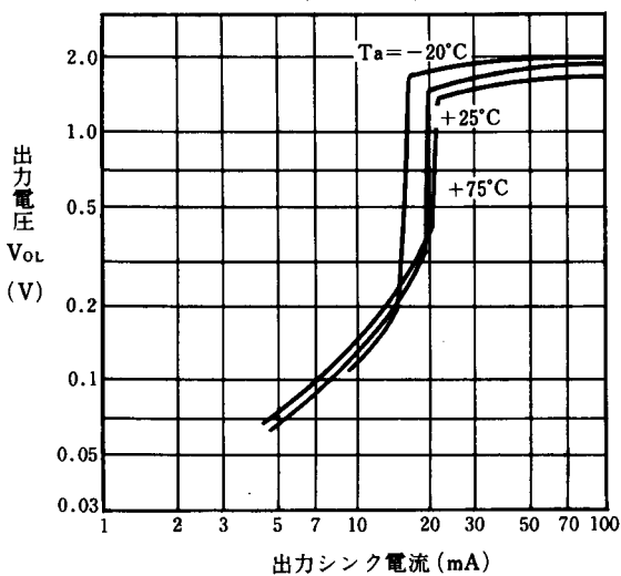
出力電圧対出力シンク電流特性例 ( V^+ = 5\text{V} )
