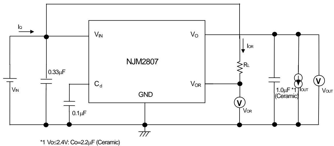
応用回路例
