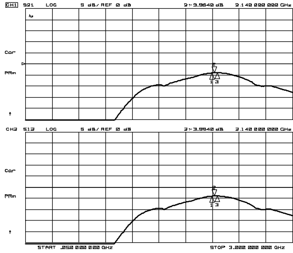
S21, S12
