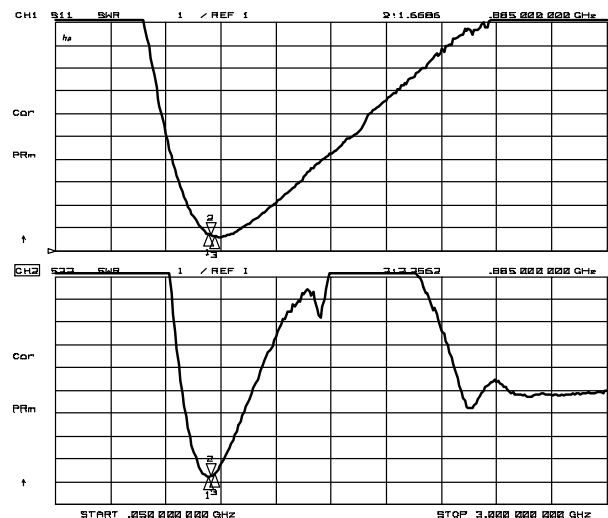
VSWR
