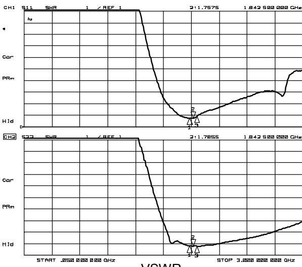
VSWR
