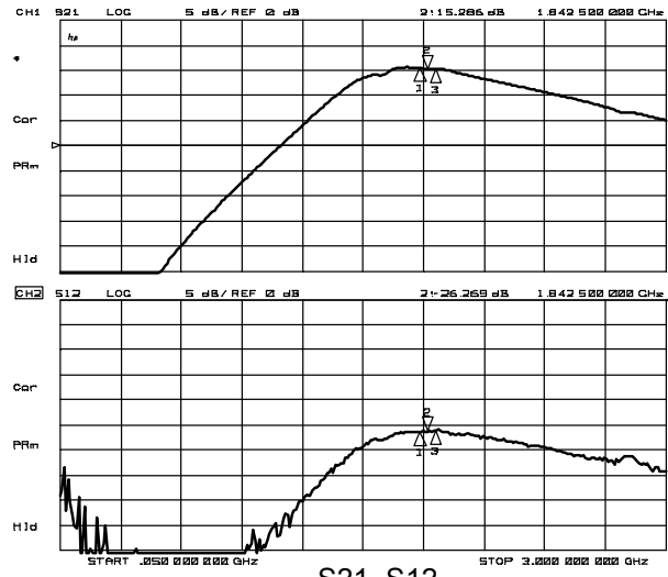
S21, S12
