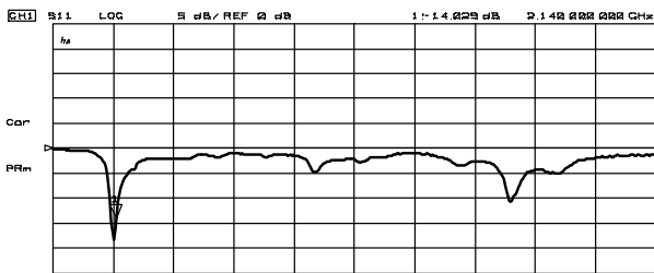
VSWR
