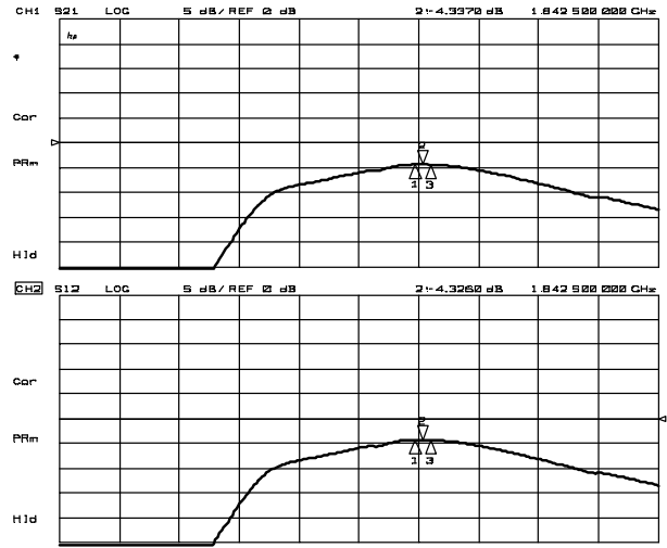
S21, S12
