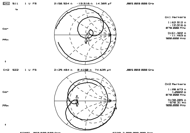
Zin, Zout
