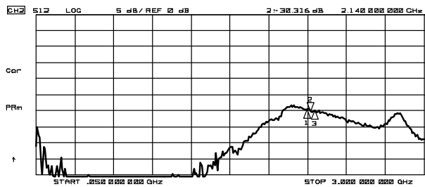
S21, S12
