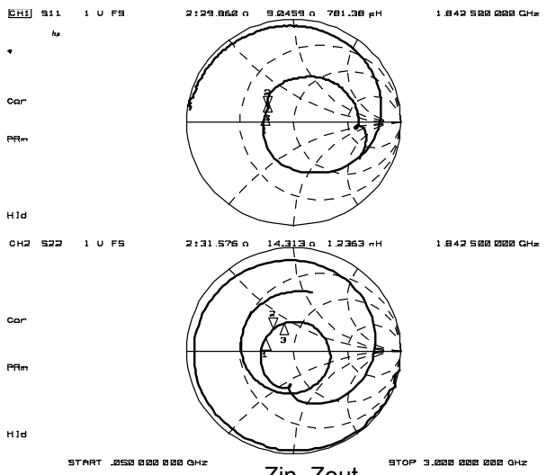
Zin, Zout
