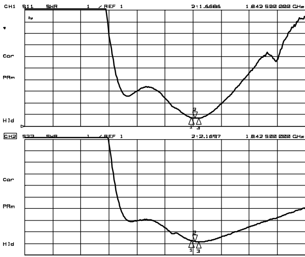
VSWR
