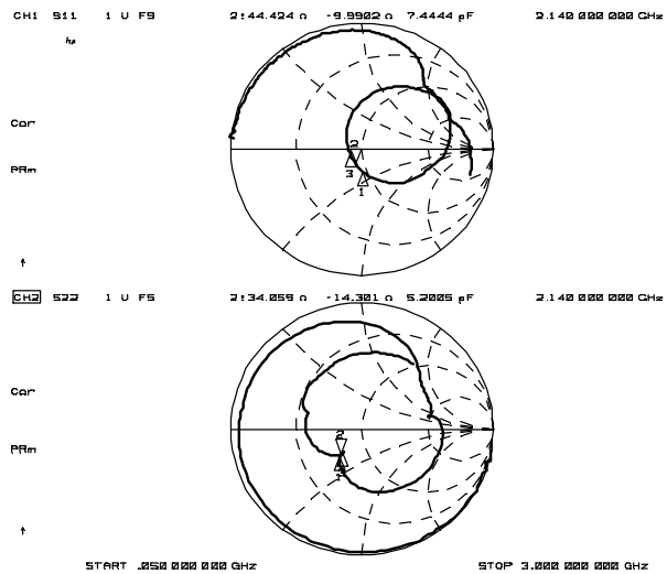
Zin, Zout
