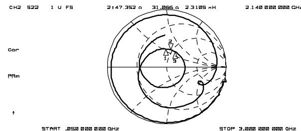
Zin, Zout
