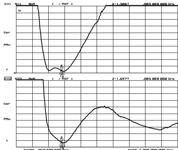
VSWR
