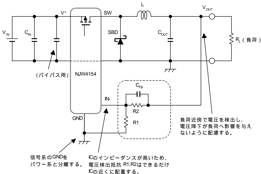
図6 降圧回路での配線例
