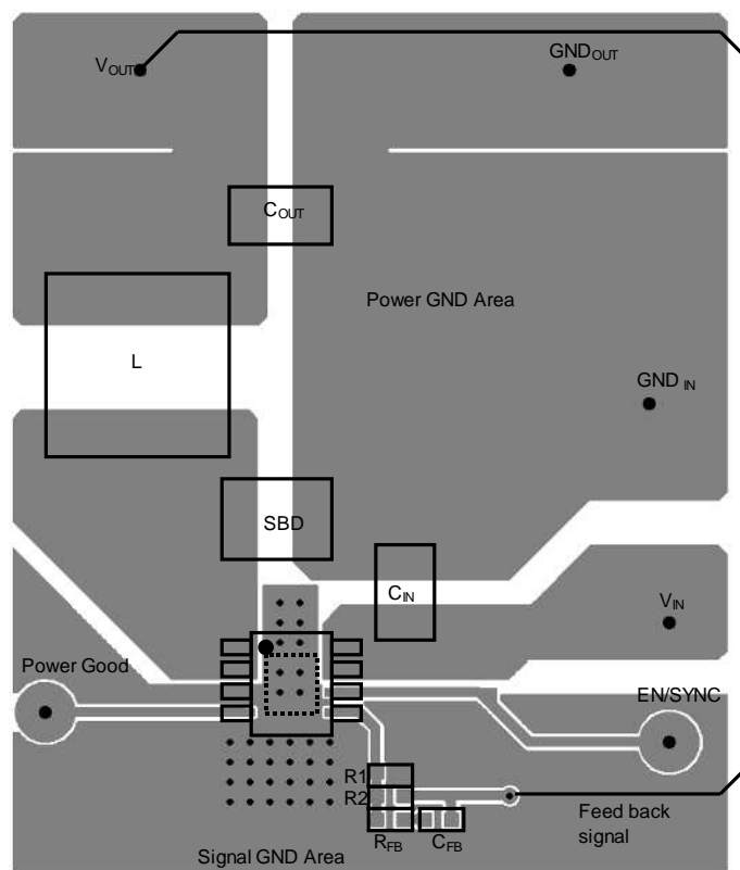
HSOP8 パッケージ
