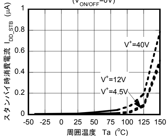
スタンバイ時消費電流温度特性例
