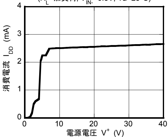
消費電流対電源電圧特性例 ( R_L =無負荷, V_{IN-}=0.5V, Ta=25^\circ C )
