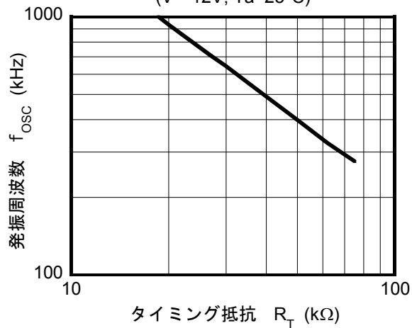
発振周波数対タイミング抵抗特性例 ( V^+=12V, Ta=25^\circ C )
