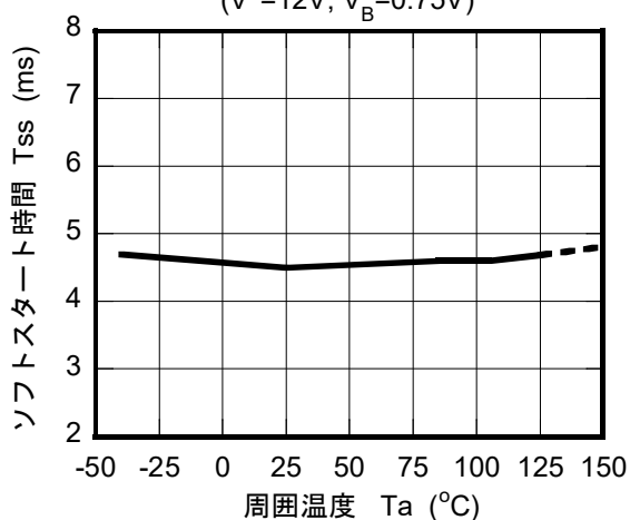
ソフトスタート時間温度特性例 ( V^+=12V , V_B=0.75V )
