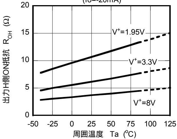
出力部(P&N) 出力H側ON抵抗温度特性例 ( I_o=-20\text{mA} )
