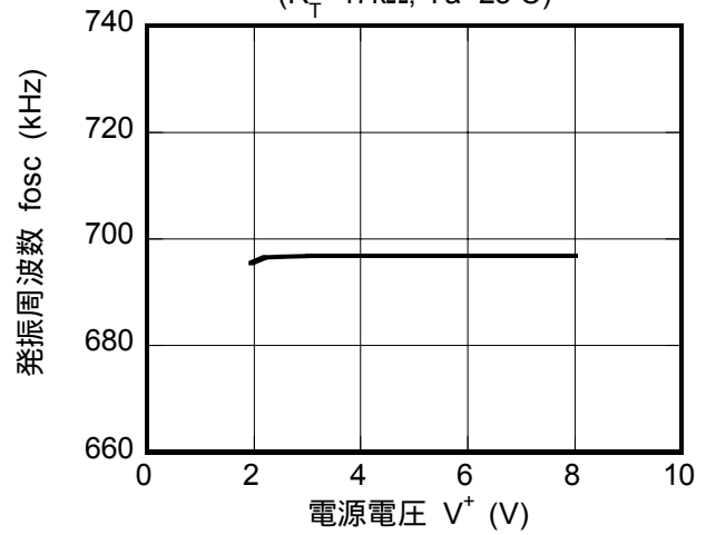
発振周波数対電源電圧特性例 ( R_T = 47k\Omega, T_a = 25^\circ C )
