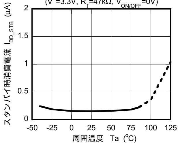
スタンバイ時消費電流温度特性例 ( V^+=3.3V , R_T=47k\Omega , V_{ON/OFF}=0V )
