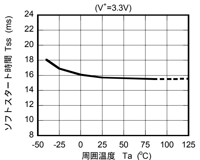
ソフトスタート時間温度特性例
