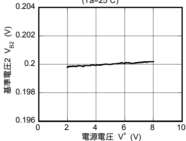
電流センスアンプ部 基準電圧2対電源電圧特性例
