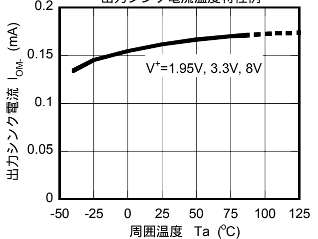
誤差増幅器, 電流センスアンプ部 出力シンク電流温度特性例
