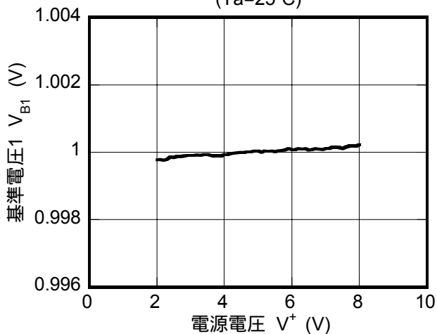
誤差増幅器部 基準電圧1対電源電圧特性例
