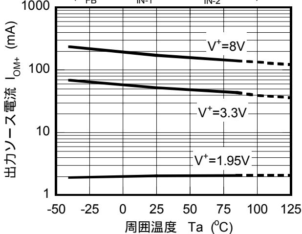
誤差増幅器部 出力ソース電流1温度特性例 ( V_{FB}=1V , V_{IN-1}=0.9V , V_{IN-2}=0.1V )
