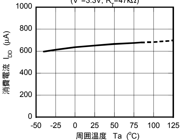
消費電流温度特性例 ( V^+=3.3V, R_f=47k\Omega )
