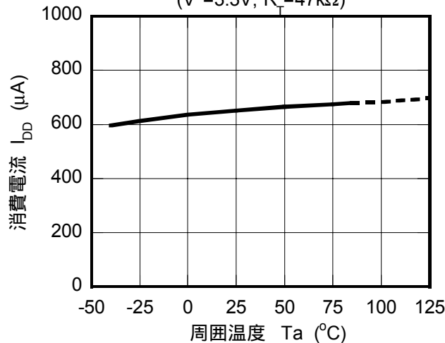
消費電流温度特性例 ( V^+=3.3V, R_f=47k\Omega )
