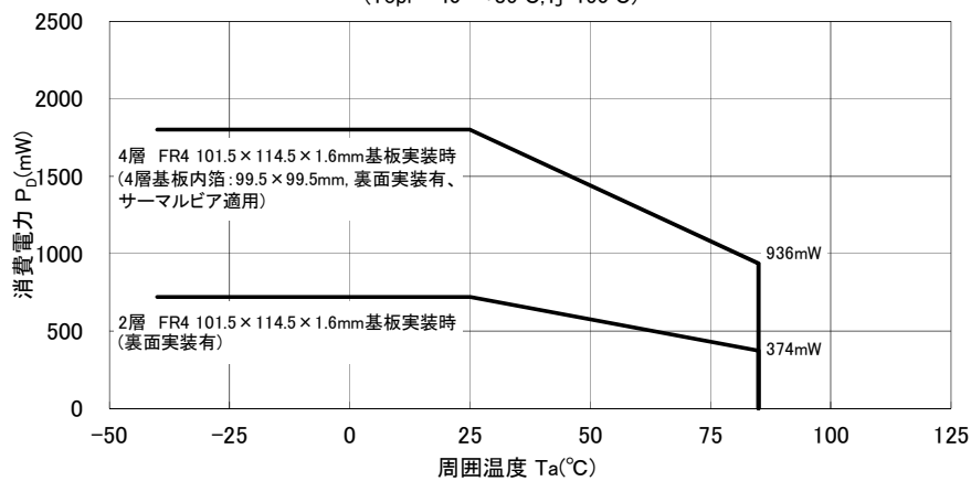
NJU7381AMJE デイレーティングカーブ ( T_{opr} = -40 \sim +85^{\circ}\text{C} , T_j = 150^{\circ}\text{C} )
