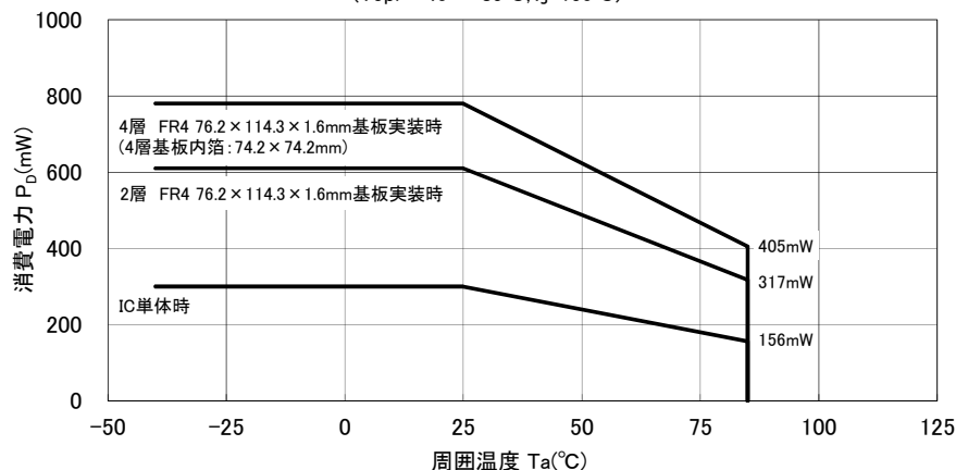
NJU7381AV デイレーティングカーブ ( T_{opr} = -40 \sim +85^{\circ}\text{C} , T_j = 150^{\circ}\text{C} )
