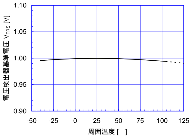
電圧検出器基準電圧 温度特性 (V+=3.3V)
