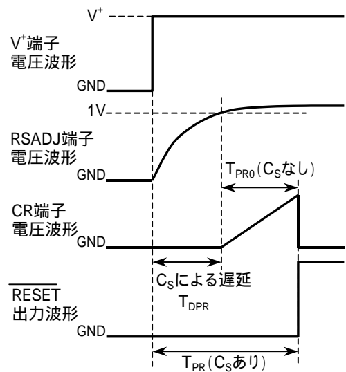
図 8. コンデンサ C_S 挿入時の各電圧波形
