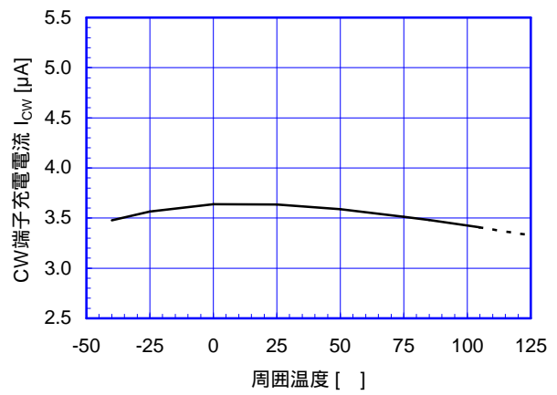
CW端子充電電流 (V+=7V)
