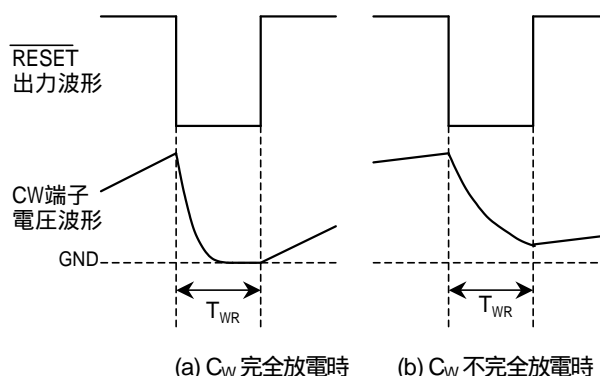
図 4. ウォッチドッグタイマリセット時間 T_{WR} と CW 端子の電圧波形
