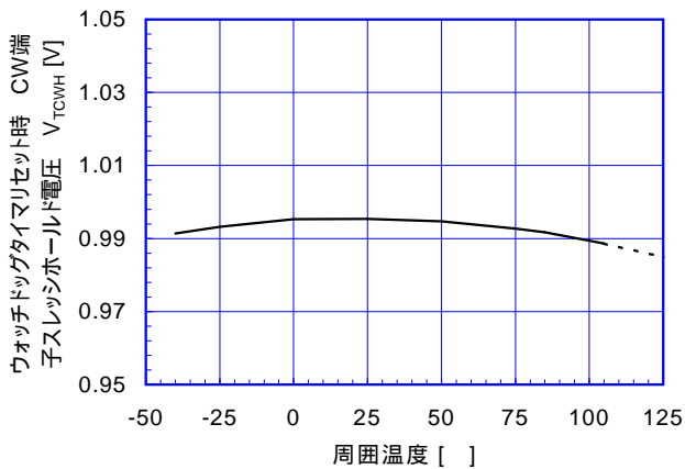
ウォッチドッグタイマリセット時CW端子スレッシュホールド電圧 温度特性 (V+=3.3V)
