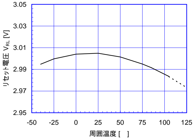
リセット電圧 温度特性 (V+=3.3V)
