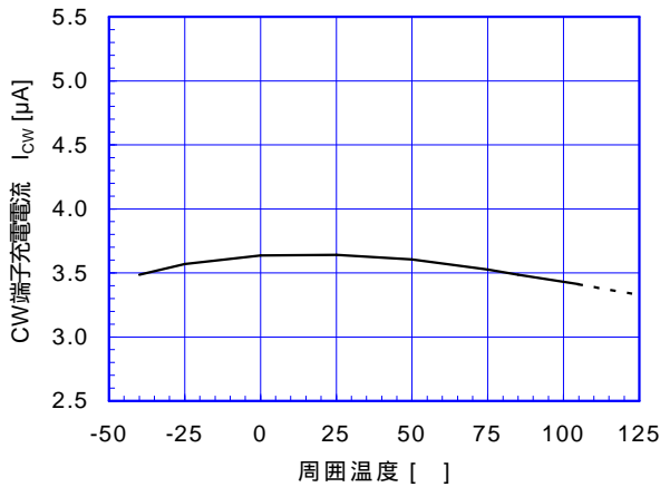
CW端子充電電流 (V+=3.3V)
