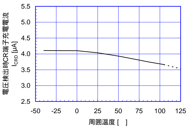
電圧検出時CR端子充電電流 温度特性 (V+=3.3V)
