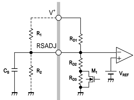
図 7. 電源ノイズに対する対応方法
