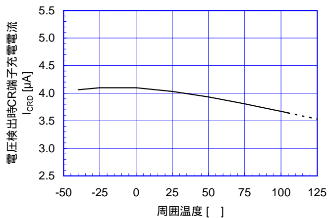
電圧検出時CR端子充電電流 温度特性 (V+=7V)
