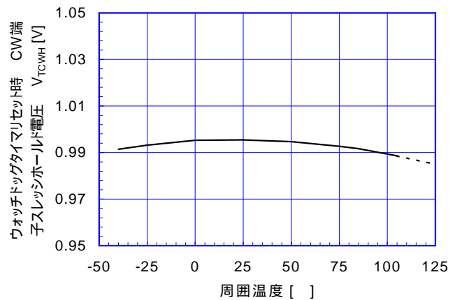
ウォッチドッグタイマリセット時CW端子スレッシュホールド電圧 温度特性 (V+=7V)
