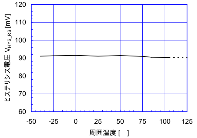
ヒステリシス電圧 温度特性 (V+=3.3V)
