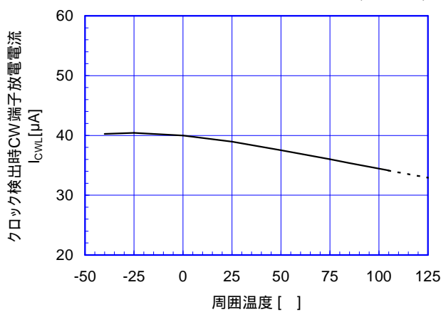
クロック検出時CW端子放電電流 温度特性 (V+=3.3V)
