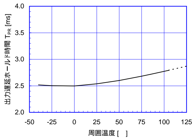
出力遅延ホールド時間 温度特性 (V+=3.3V)
