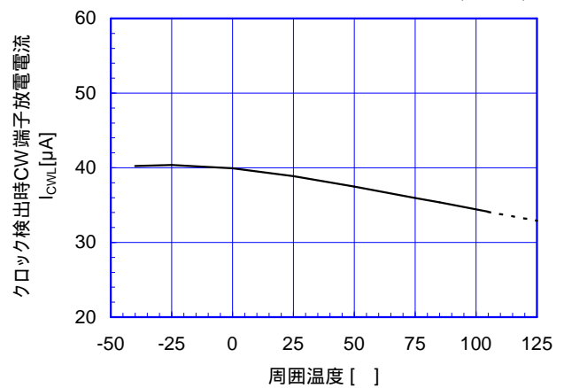
クロック検出時CW端子放電電流 温度特性 (V+=7V)
