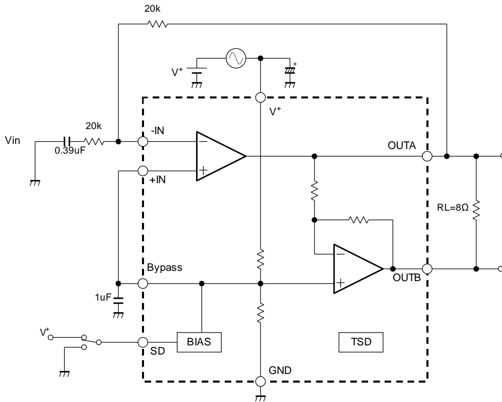
測定回路 3 (PSRR)
