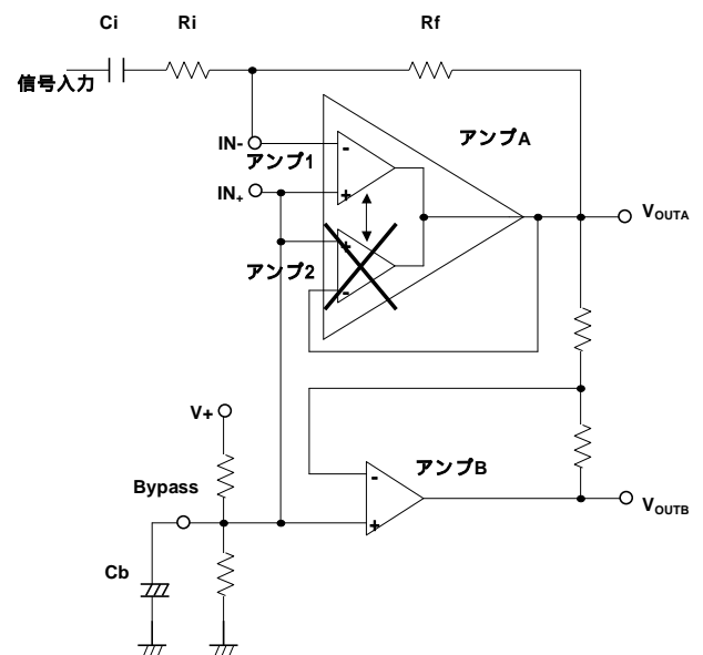
図 3 反転アンプ動作時
