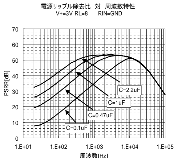
図 10 PSRR 対 C_b ( V^+=3V )
