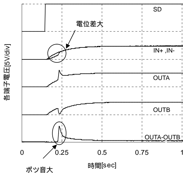
図5 R_f=100k 時の各端子電圧
