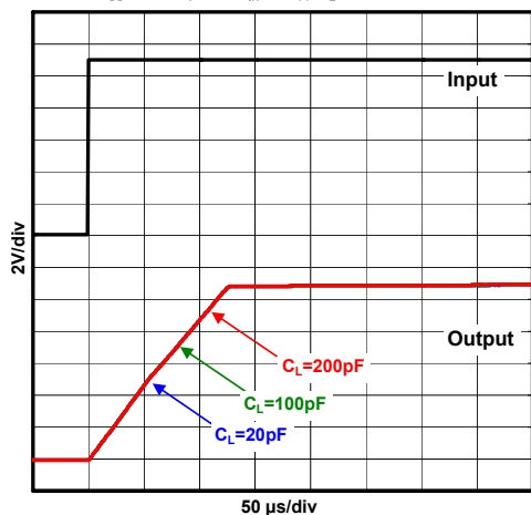
過渡応答特性例 V_{DD}=15V, G_V=0dB, V_{IN}=11V_{pp}, R_L=10k\Omega, T_a=25^\circ C
