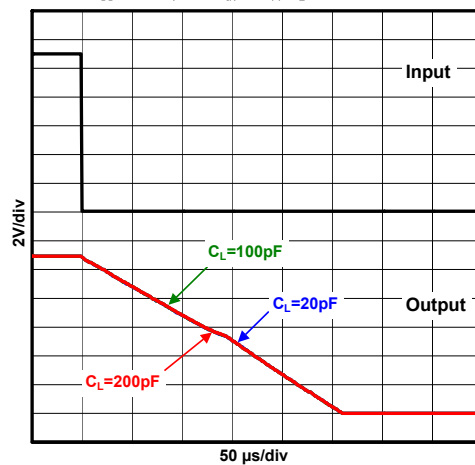
過渡応答特性例 V_{DD}=15V, G_V=0dB, V_{IN}=11V_{pp}, R_L=10k\Omega, T_a=25^\circ C
