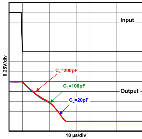
過渡応答特性例 V_{DD}=5V, G_V=0dB, V_{IN}=1V_{pp}, R_L=10k\Omega, T_a=25^\circ C
