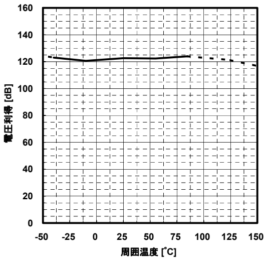
電圧利得 対 周囲温度特性例 V_{DD}=10V, R_L=10k\Omega, V_o=V_{DD}/2\pm 3V
