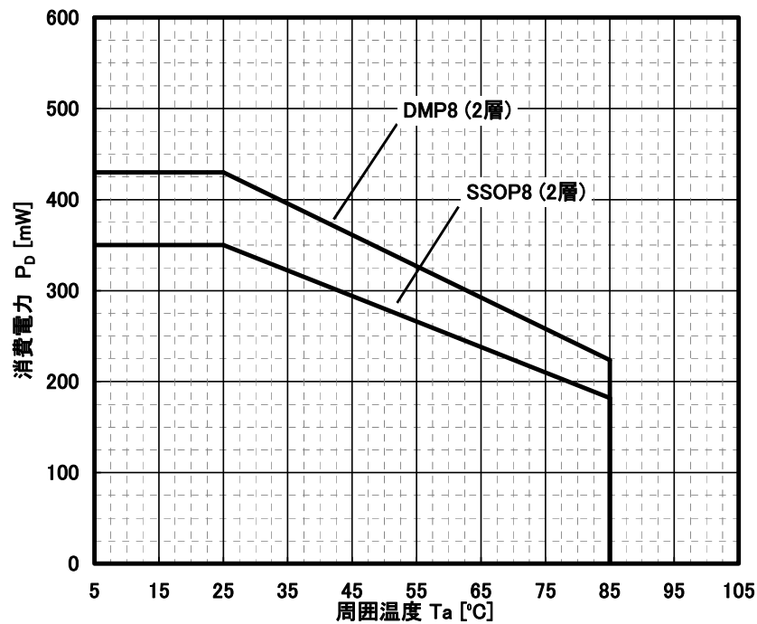
図 1. 消費電力 対 周囲温度特性例
