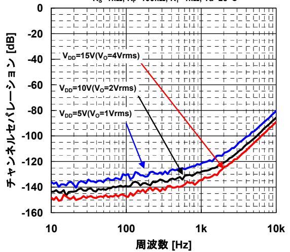
チャンネルセレーション 対 周波数特性 R_s=1k\Omega, R_f=100k\Omega, R_i=1k\Omega, T_a=25^\circ C
