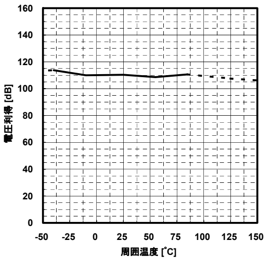
電圧利得 対 周囲温度特性例 V_{DD}=5V, R_L=10k\Omega, V_o=V_{DD}/2\pm 1.5V
