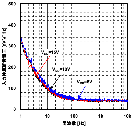
入力換算雑音電圧 対 周波数特性 R_s=1k\Omega, R_f=10k\Omega, T_a=25^\circ C
