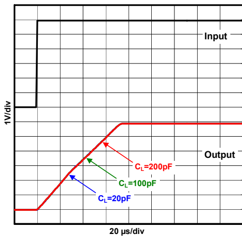
過渡応答特性例 V_{DD}=10V, G_V=0dB, V_{IN}=6V_{pp}, R_L=10k\Omega, T_a=25^\circ C
