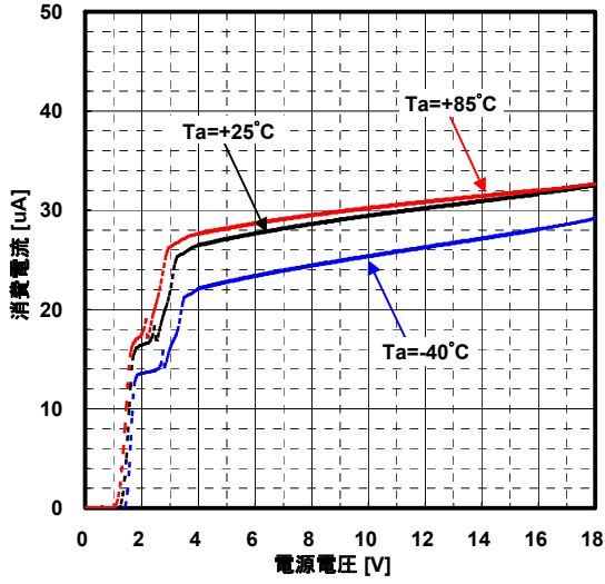
消費電流 対 電源電圧 特性例 G_V=0\text{dB}, V_{ICM}=V_{DD}/2
