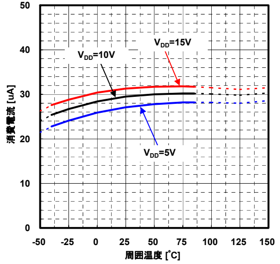
消費電流 対 周囲温度 特性例 G_V=0\text{dB}, V_{ICM}=V_{DD}/2
