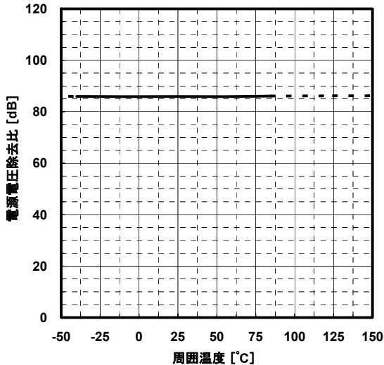
電源電圧除去比 対 周囲温度 特性例 V_{DD}=4\text{V to }16\text{V}, V_{ICM}=V_{DD}/2
