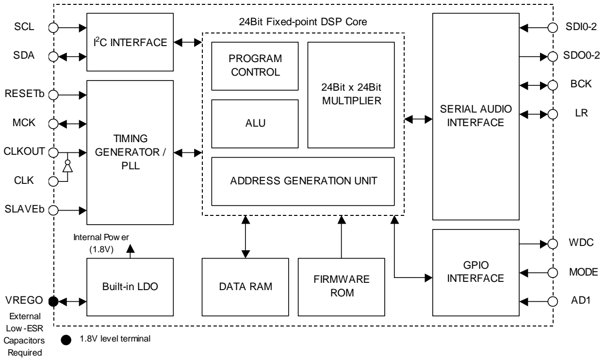
図1 NJU26124 ハードウェアブロック図
