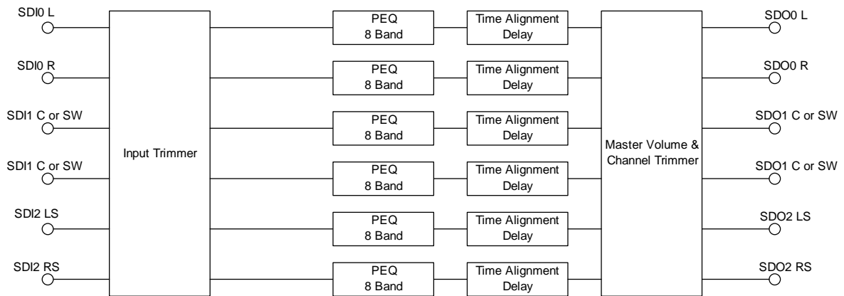
図2-3 PEQ + Time Alignment Delay経路ブロック図
