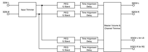
図2-4-4 Output : 4ch (2ch)
