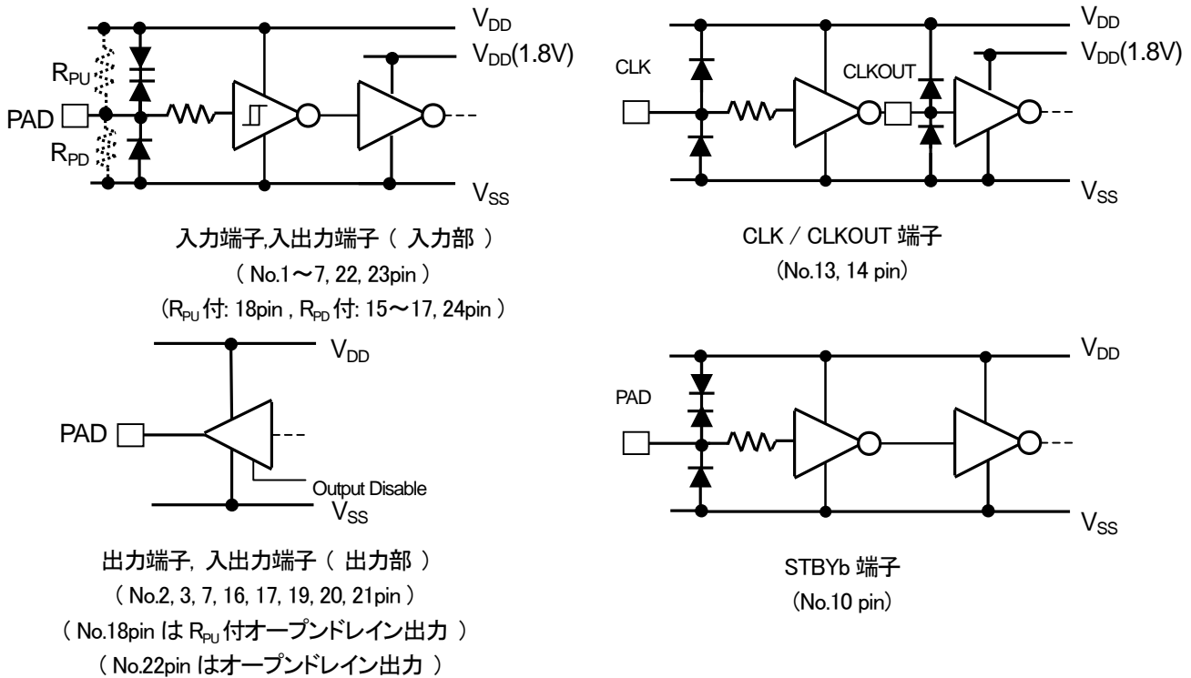
図 4 NJU26124 入出力等価回路図
