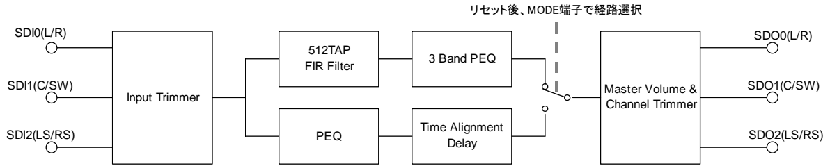
図2-1 NJU26124機能ブロック図
