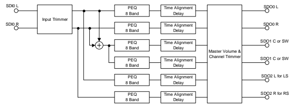
図2-4-6 Output : 5.1ch (3.1ch)
