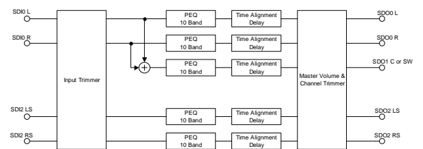
図2-6-2 Output : 4.1ch or 5ch
