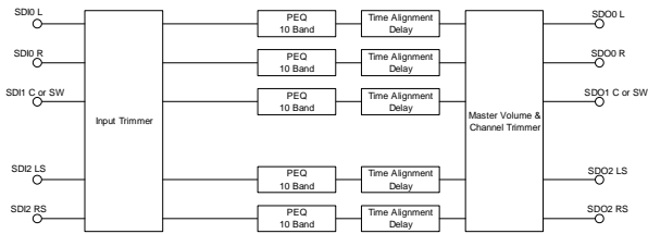
図2-7-1 Output : 4.1ch or 5ch
