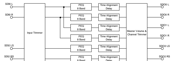
図2-6-4 Output : 6ch (4ch)
