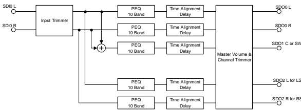
図2-4-5 Output : 4.1ch or 5ch (2.1ch or 3ch)
