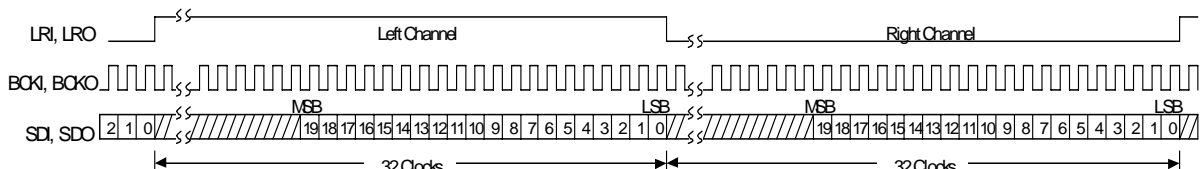
図 6-6 Right-Justified Data Format 64fs, 20bit Data
