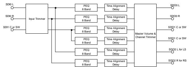
図2-5-4 Output : 5.1ch (3.1ch)
