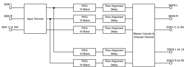
図2-5-3 Output : 4.1ch or 5ch (2.1ch or 3ch)
