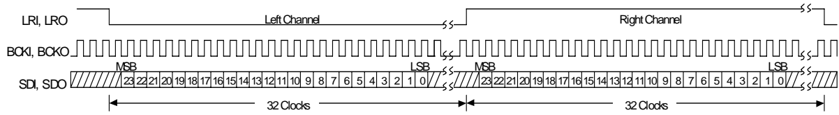
図 6-1 I 2 S Data Format 64fs, 24bit Data
