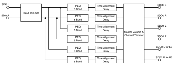
図2-4-7 Output : 6ch (2ch)
