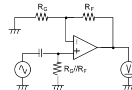
測定回路
