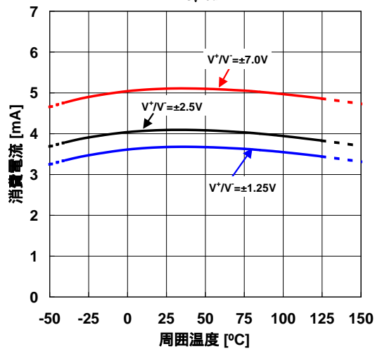
消費電流 対 周囲温度特性例 (電源電圧) G_V=0\text{dB}
