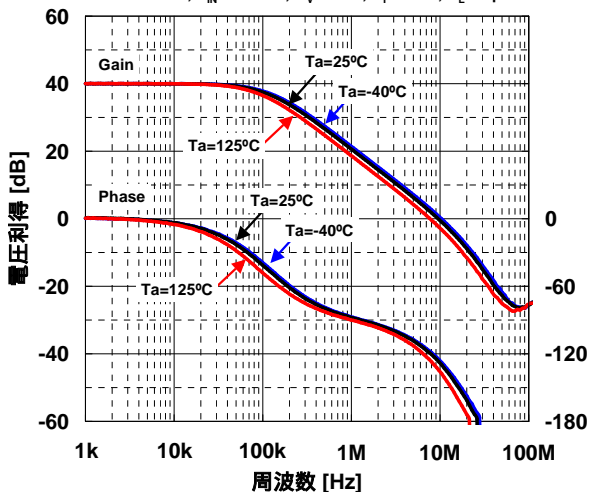
40dB 電圧利得/位相 对 周波数特性例 (周囲温度) V^+V^- = \pm 2.5\text{V} , V_{IN} = -30\text{dBm} , G_V = 40\text{dB} , R_F = 10\text{k}\Omega , C_L = 10\text{pF}
