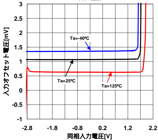
入力オフセット電圧 対 同相入力電圧特性例 (周囲温度) V^*/V = \pm 2.5\text{V}
