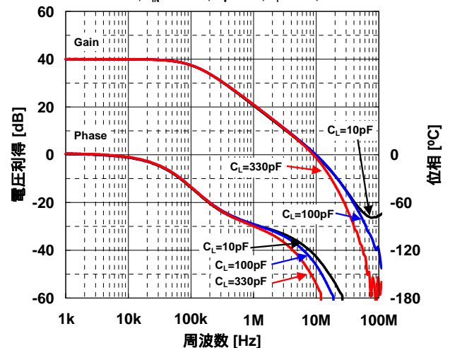
40dB 電圧利得/位相 对 周波数特性例 (負荷容量) V^+V^- = \pm 2.5\text{V} , V_{IN} = -30\text{dBm} , G_V = 40\text{dB} , R_F = 10\text{k}\Omega , T_a = 25^\circ\text{C}
