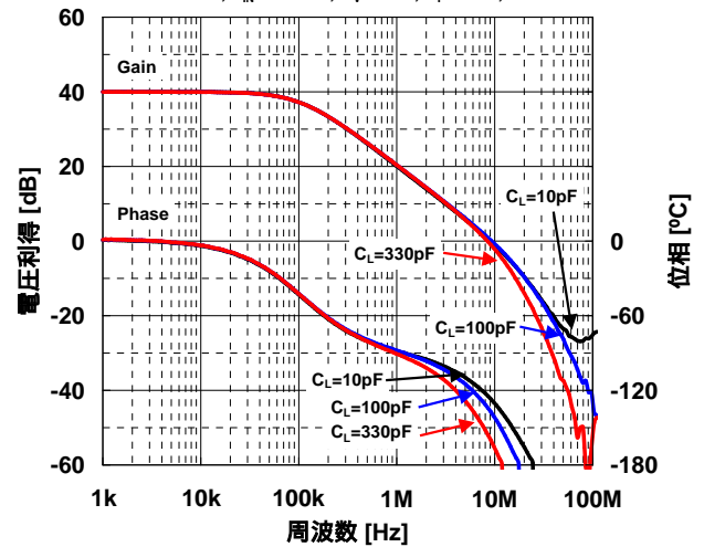
40dB 電圧利得/位相 对 周波数特性例 (負荷容量) V^+V^- = \pm 1.25\text{V} , V_{IN} = -30\text{dBm} , G_V = 40\text{dB} , R_F = 10\text{k}\Omega , T_a = 25^\circ\text{C}
