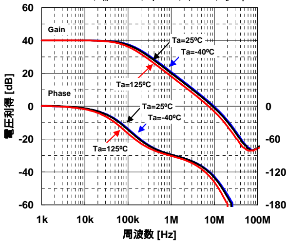
40dB 電圧利得/位相 对 周波数特性例 (周囲温度) V^+V^- = \pm 1.25\text{V} , V_{IN} = -30\text{dBm} , G_V = 40\text{dB} , R_F = 10\text{k}\Omega , C_L = 10\text{pF}
