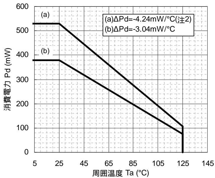
ディレーティングカーブ 特性例 (DMP8)
