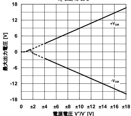
最大出力電圧 对 電源電圧 特性例 R_L = 2k\Omega, T_a = 25^\circ C
