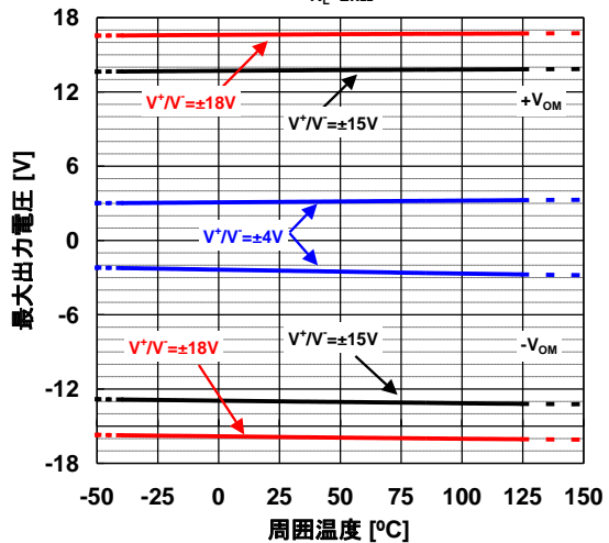
最大出力電圧 对 周围温度 特性例 R_L = 2k\Omega
