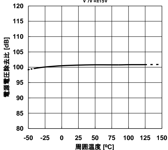
電源電圧除去比 对 周围温度 特性例 V^*/V = \pm 15V
