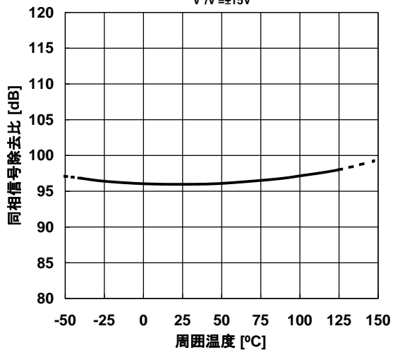
同相信号除去比 对 周围温度 特性例 V^*/V = \pm 15V
