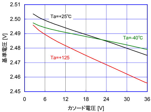
NJM431-Z 基準電圧対カソード電圧
