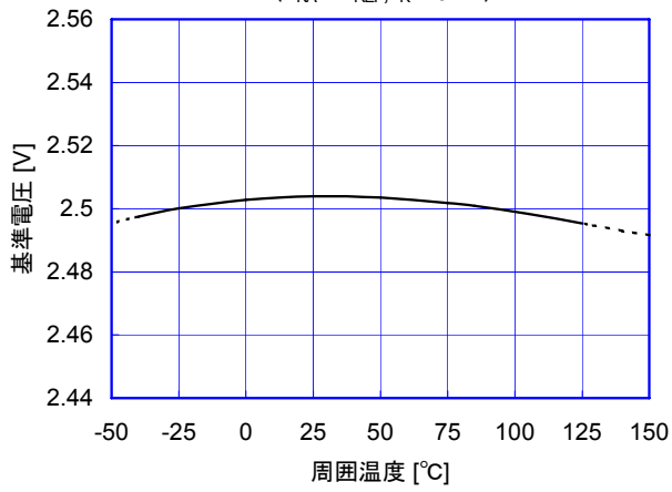
NJM431-Z 基準電圧温度特性
