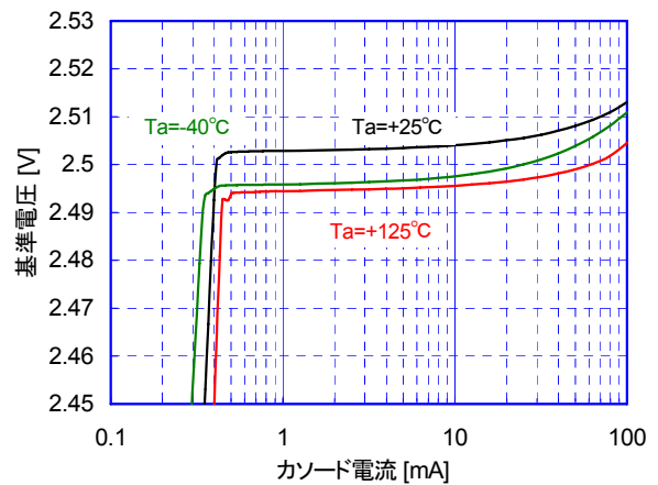
NJM431-Z 基準電圧対カソード電流
