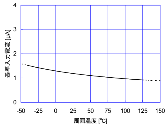
NJM431-Z 基準入力電流温度特性
