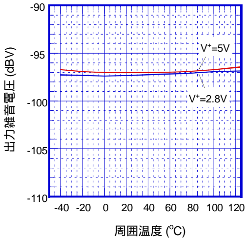
出力雑音電圧 对 周囲温度特性例 ( RL = 32\Omega, A\text{-Weighted} )
