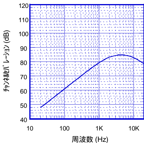
チャンネルレージョン 対 周波数特性例 ( V^+=5V, f=1\text{kHz}, R_L=32\Omega )
