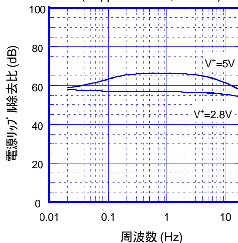
電源リップル除去比 対 周波数特性例 ( V_{\text{ripple}}=-20\text{dBV}, R_L=32\Omega )
