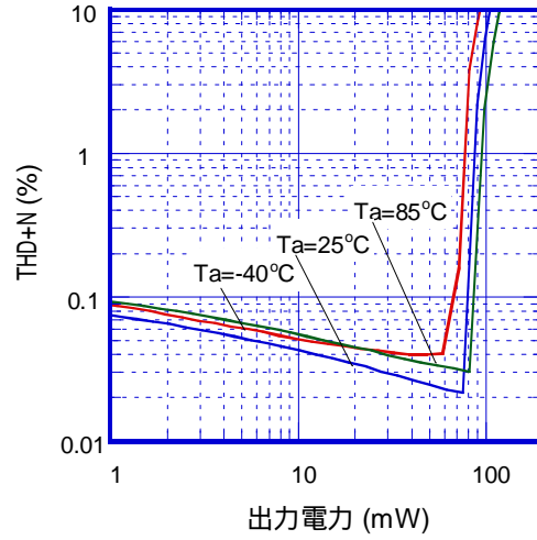
THD+N 对 出力電力特性例 ( V_+ = 5V, f = 1KHz, RL = 16\Omega )
