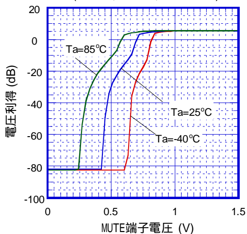
電圧利得 対 MUTE端子電圧特性例 ( V^+=5V, f=1\text{kHz}, V_{\text{in}}=-6\text{dBV} )
