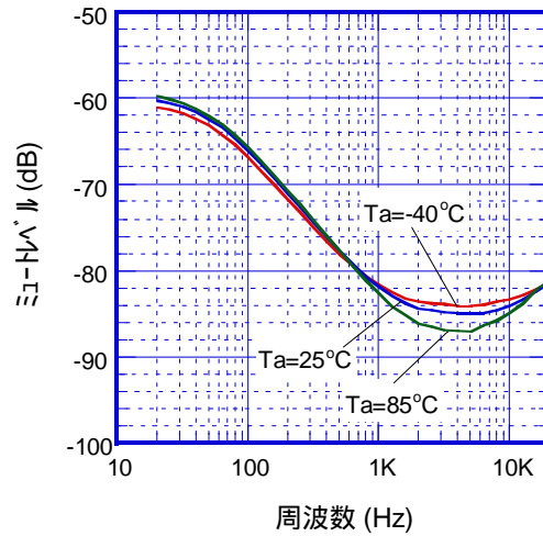
ミュートル対 周波数特性例 ( V_+ = 5V, Vin = -6dBV, RL = 32\Omega )
