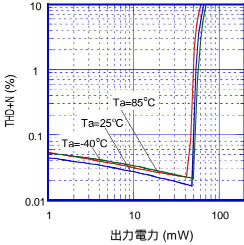
THD+N 对 出力電力特性例 ( V_+ = 5V, f = 1KHz, RL = 32\Omega )
