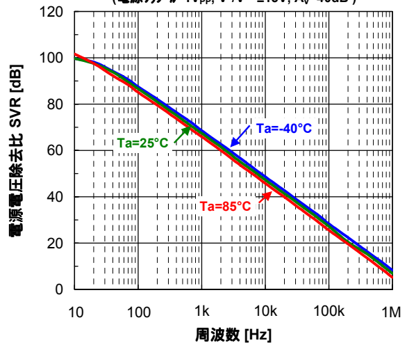
電源電圧除去比(負電源側) - 周波数 (電源リップル = 1V_{PP} , V^+/V^- = \pm 15V , A_V = 40dB )
