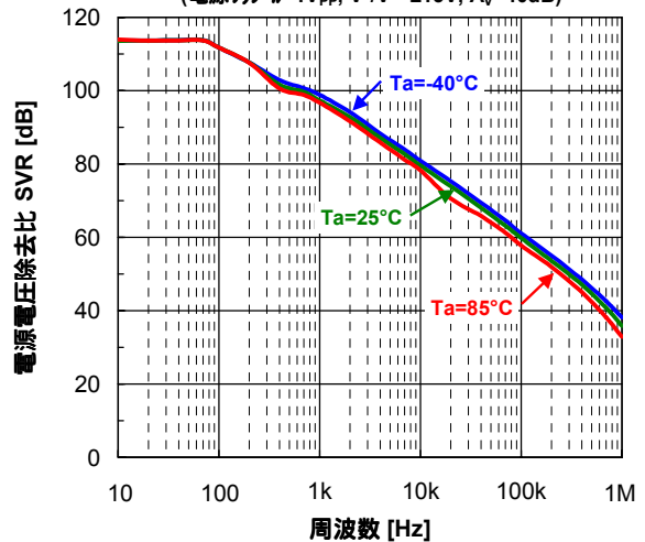
電源電圧除去比(正電源側) - 周波数 (電源リップル = 1V_{PP} , V^+/V^- = \pm 15V , A_V = 40dB )
