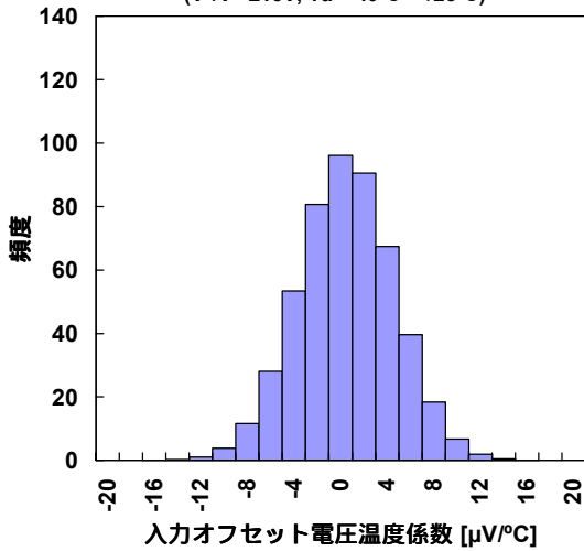
入力オフセット電圧温度係数分布 ( V^+/V^-=\pm 15V , T_a=-40^\circ C + 25^\circ C )
