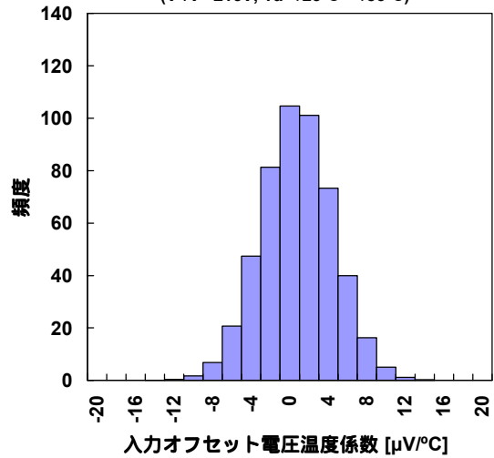
入力オフセット電圧温度係数分布 ( V^+/V^-=\pm 15V , T_a=+25^\circ C + 85^\circ C )
