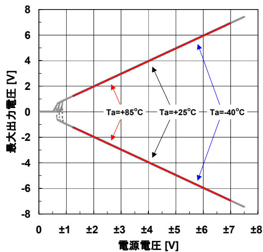
最大出力電圧 対 電源電圧特性例 (周囲温度・ R_L=10k\Omega ) G_V=OPEN, R_L=10k\Omega
