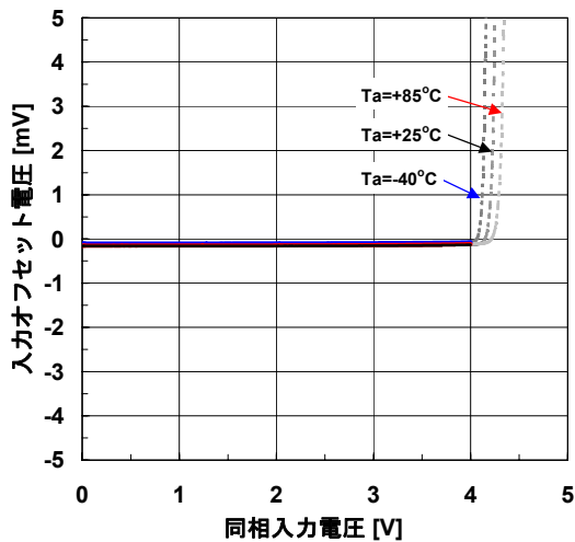
入力オフセット電圧 対 同相入力電圧特性例 (周囲温度・ V^+=5\text{V} )
