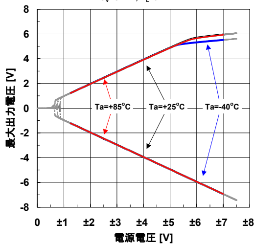
最大出力電圧 対 電源電圧特性例 (周囲温度・ R_L=5k\Omega ) G_V=OPEN, R_L=5k\Omega
