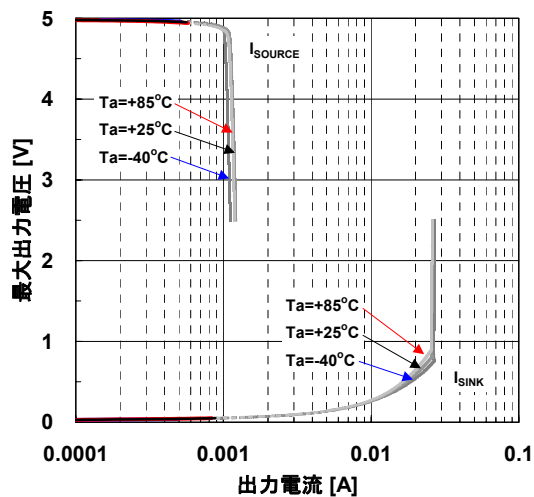
最大出力電圧 対 出力電流特性例 (周囲温度・ V^+=5V ) V^+=5V, G_V=OPEN
