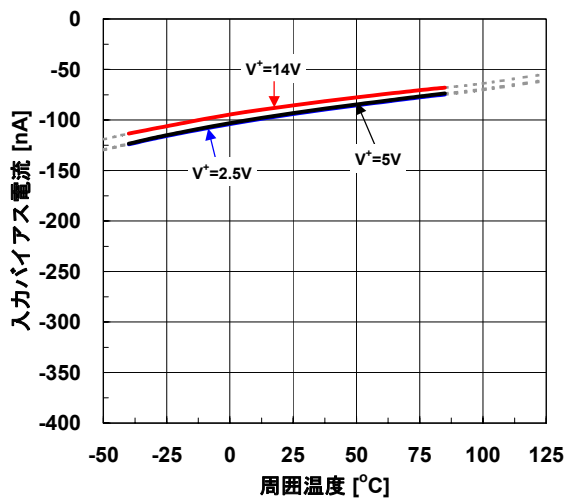
入力バイアス電流 対 周囲温度特性例 (電源電圧) R_L=10k\Omega
