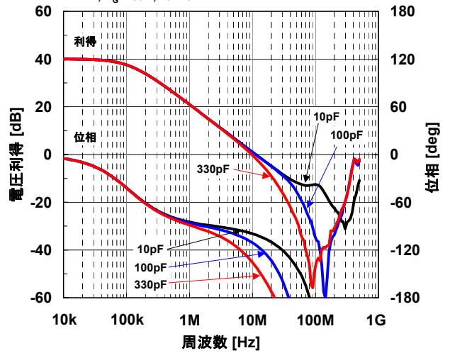
位相余裕 対 負荷容量特性例 (周囲温度)
