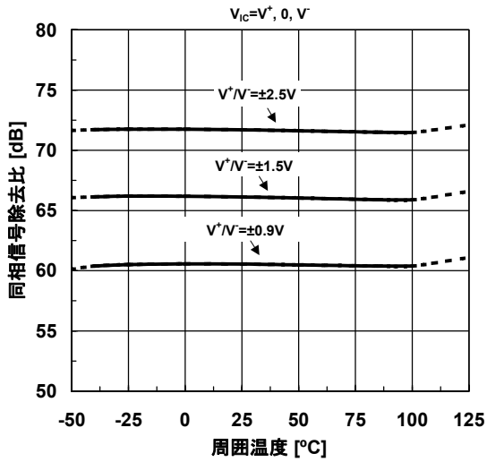
同相信号除去比 对 周围温度特性例
