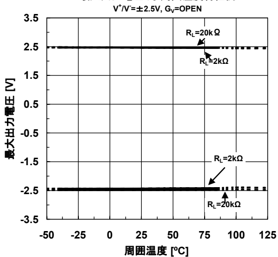
最大出力電圧 对 周围温度特性例
