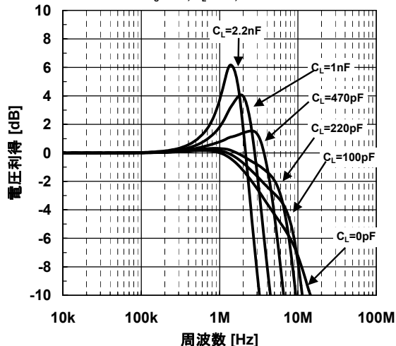
ホールドアップのピーク利得特性例
