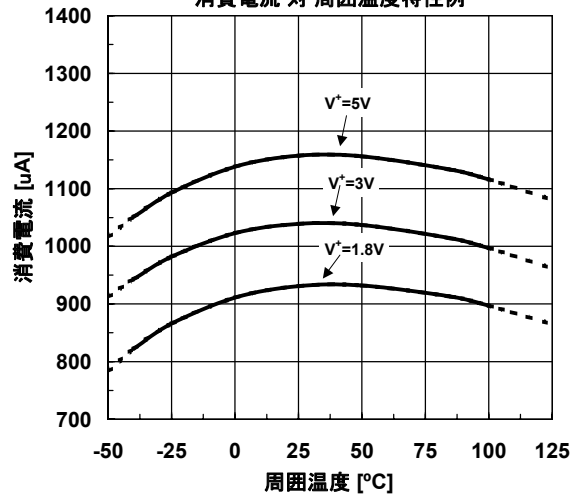
消費電流 対 周囲温度特性例
