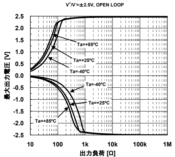
最大出力電圧 对 出力負荷特性例
