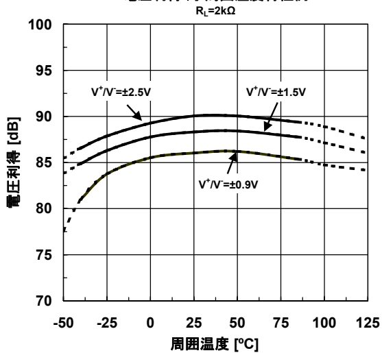
電圧利得 对 周围温度特性例
