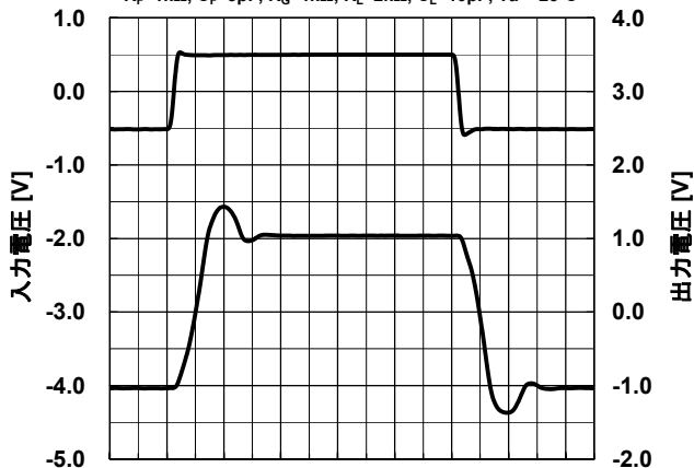
時間 10ns/div
