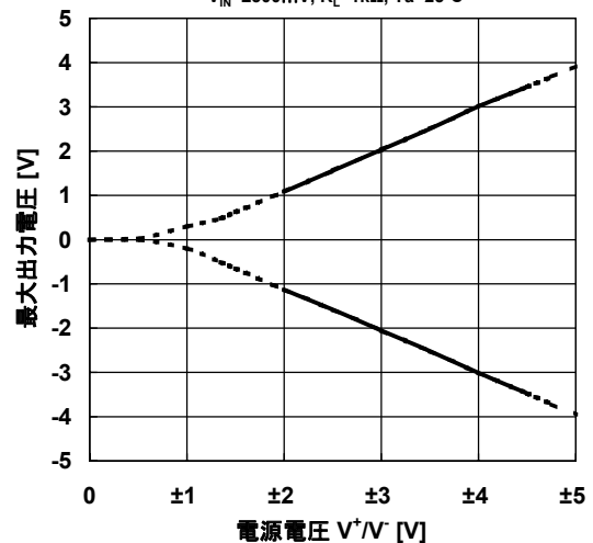
最大出力電圧 対 電源電圧 特性例
