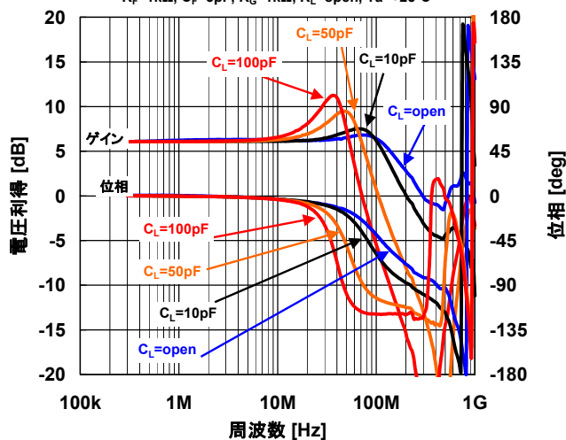
6dB電圧利得 对周波数特性例 (負荷容量)
