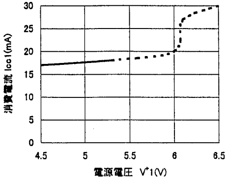
消費電流対電源電圧特性例 ( V^2=3V , 無信号時)
