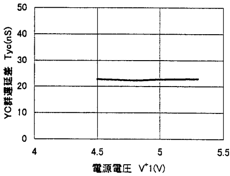
YC相对群遅延对電源電圧特性例 ( V^2=3V )
