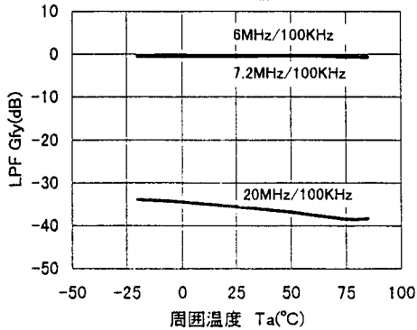
LPF対周囲温度特性例 (V'1=4.8V, V'2=3.0V, YIN=100mVpp)
