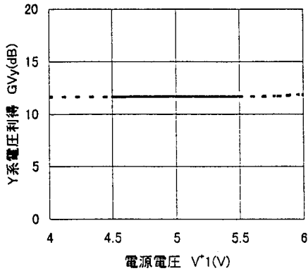
Y系電圧利得対電源電圧利得特性例 ( V^2=3V )
