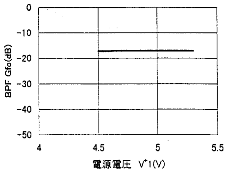
BPF对電源電圧特性例 ( V^2=3V, 500KHz/4MHz )
