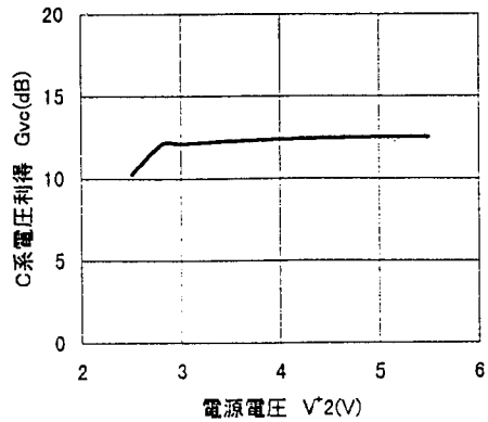
C系電圧利得対電源電圧 ( V^1=4.8V )
