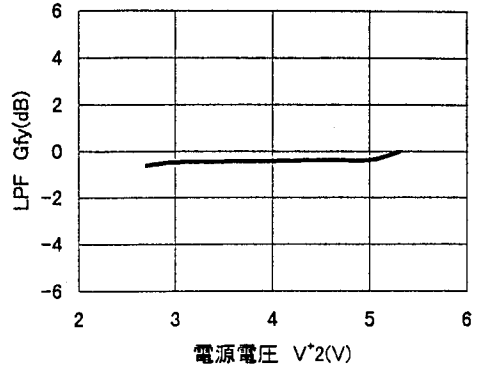
LPF对電源電圧特性例 ( V^1=4.8V, 6MHz/100kHz )
