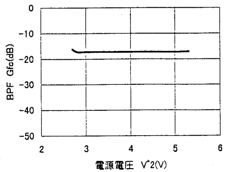
BPF对電源電圧特性例 ( V^1=4.8V, 500KHz/4MHz )
