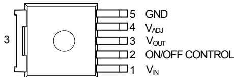
NJM2387ADL3
