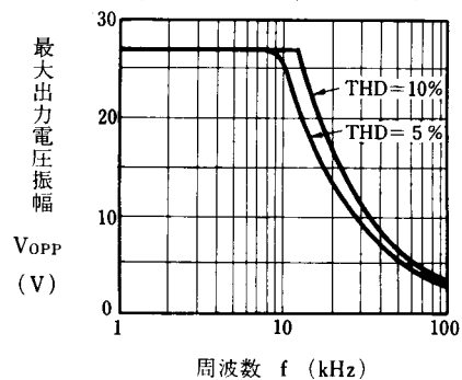
最大出力電圧周波数特性例 ( V^+/V^- = \pm 15V , T_a = 25^\circ C )
