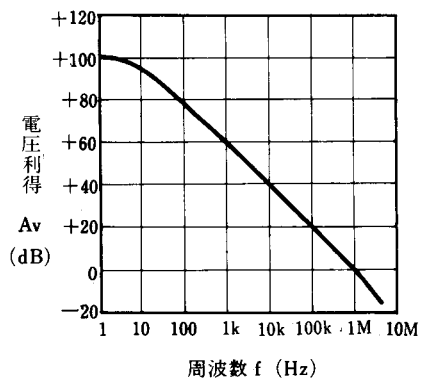
電圧利得周波数特性例 ( V^+/V^- = \pm 15V , T_a = 25^\circ C )
