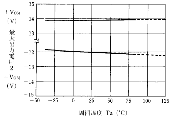
最大出力電圧 2 温度特性例 ( V^+/V^- = \pm 15V, R_L = 2k\Omega )
