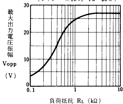
最大出力電圧振幅対負荷特性例 ( V^+/V^- = \pm 15V , T_a = 25^\circ C )
