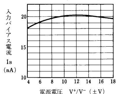
入力バイアス電流対電源電圧特性例 ( R_s = 10k\Omega , T_a = 25^\circ C )
