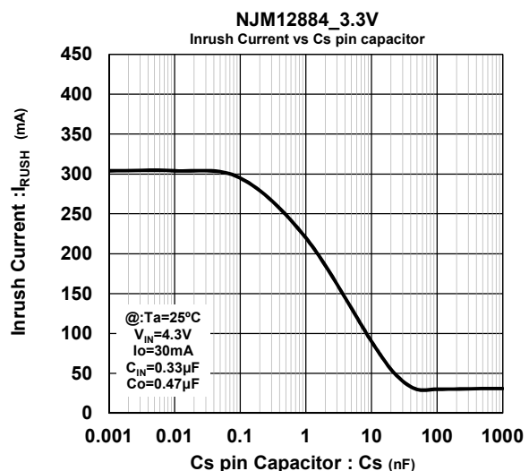
突入電流 対 C_S 端子容量特性例
