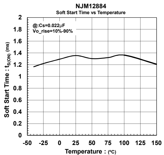
ソフトスタート時間(0.022 \mu F) 対 温度特性
