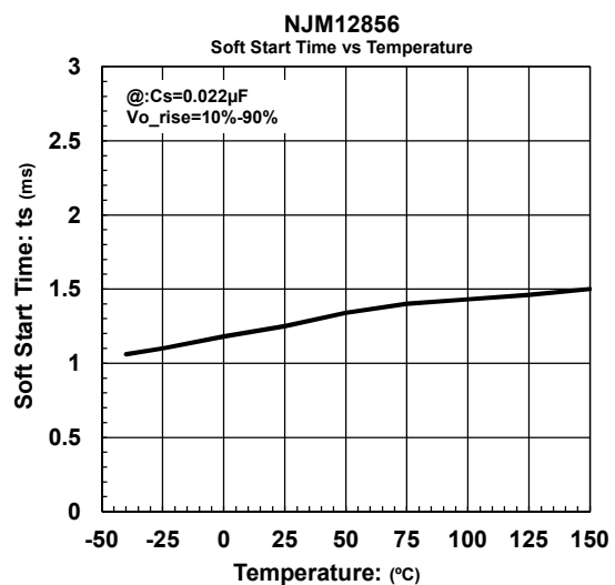
ソフトスタート時間(0.022µF) 対 温度特性
