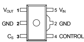
NJM12856U2
