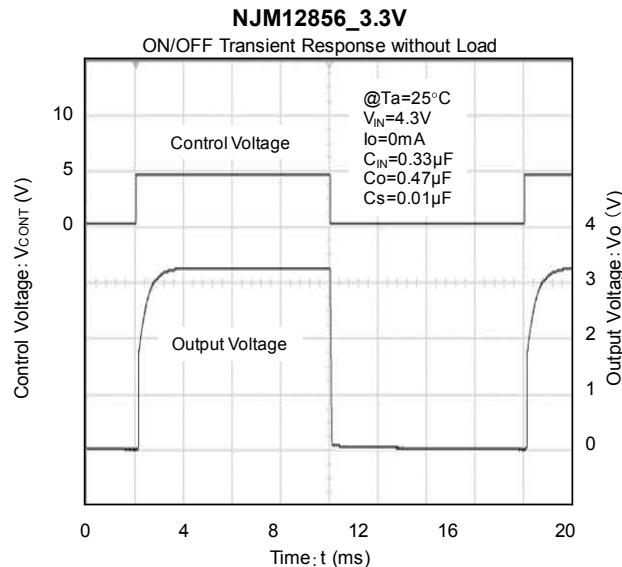
ディスチャージ機能による出力電圧立ち下り波形
