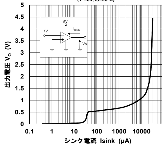
出力電圧 対 シンク電流 特性例 ( V^+=5\text{V} , T_a=25^\circ\text{C} )
