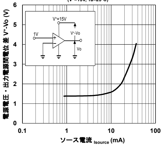
ソース電流 特性例 ( V^+=15\text{V} , T_a=25^\circ\text{C} )
