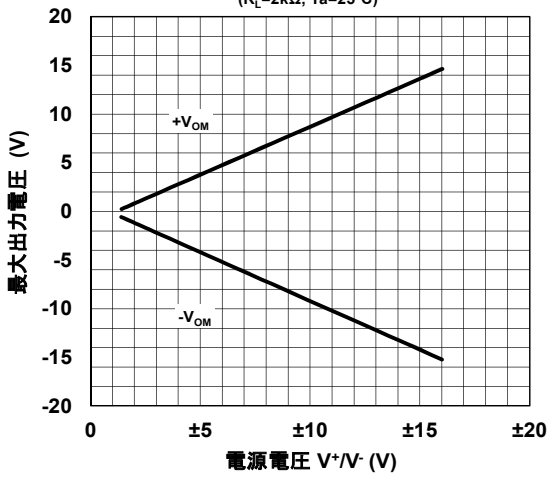
最大出力電圧 対 両電源電圧 特性例 ( R_L=2k\Omega , T_a=25^\circ\text{C} )
